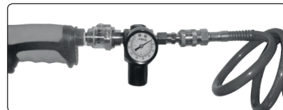
Abb. 9, Anschlussschema
