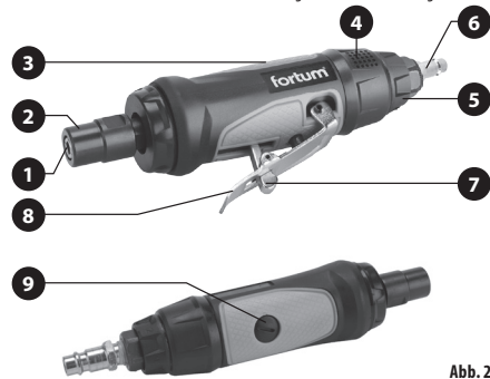
Abb.2: Position-Beschreibung
