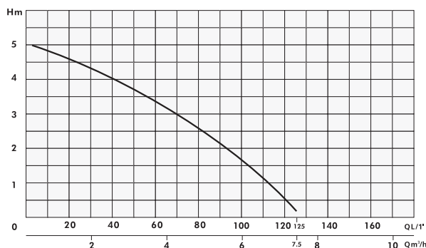
1. ábra A folyadék-áramlás ( \text{m}^3/\text{óra} ) függvénye a nyomómagasságtól.
